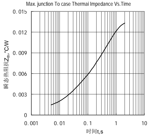
Fig.2 结至壳瞬态热阻抗曲线
